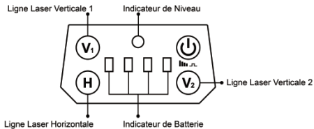
Interface pour Batterie de Type C
